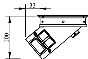
Dimensioni d'ingombro sotto piano (mm) Overall dimension under the top (mm)
